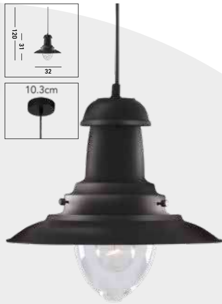
4301BK FISHERMAN Pendant Black Metal & Glass
